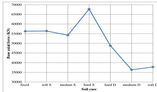
ii) Base axial force
