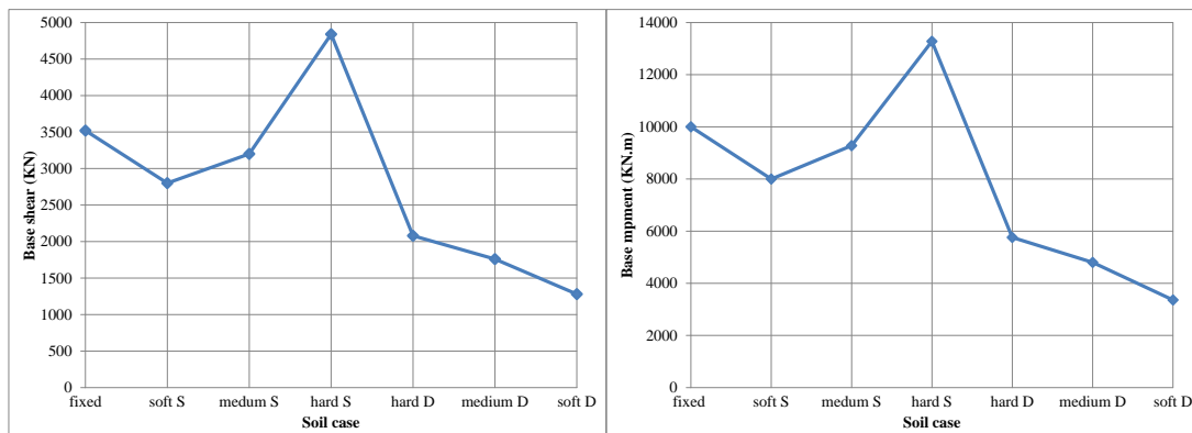
i) Base Shear
